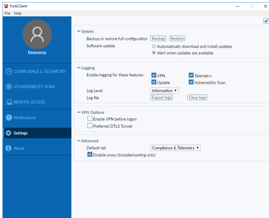
Figura 13 Pantalla Principal de Configuración VPN
